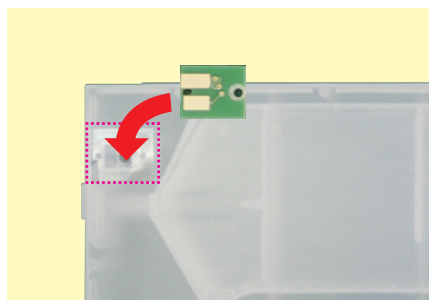
①カートリッジにチップを取付け
